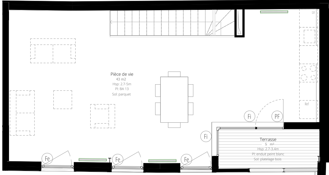
Plan R+2
